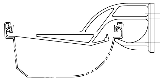
軒樋の差し替え
