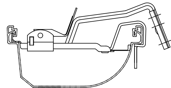
軒樋の差し替え
