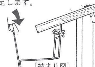
【納まり図】
