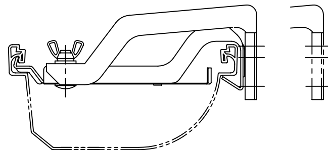
軒樋の差し替え
