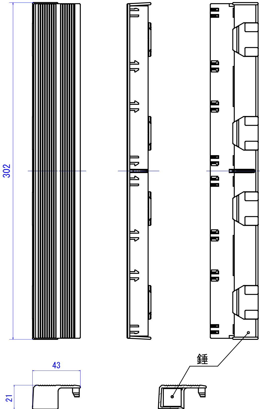
断面図
